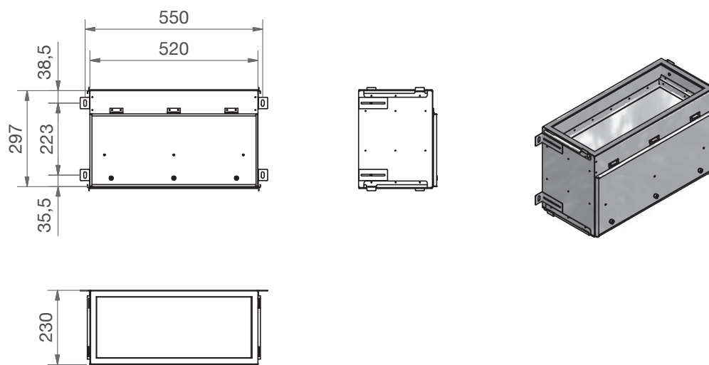
Filtri korpus
